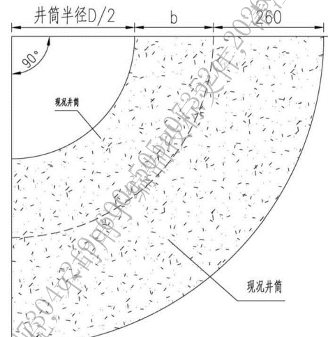
(a) 检查井加固设计图
